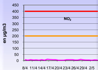
Evolution des maxima horaires en dioxyde d'azote
