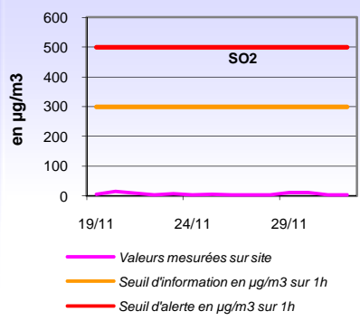
Evolution des maxima horaires en dioxyde de soufre
