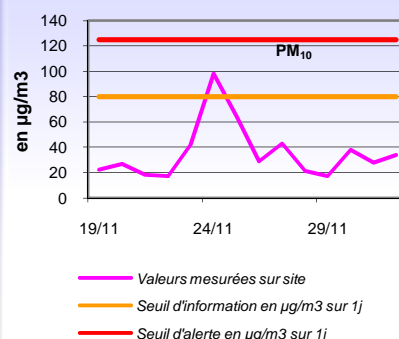
Evolution des moyennes journalières en aérosols (matière en suspension de diamètre <10 µm)
