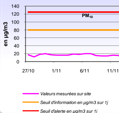
Evolution des moyennes journalières en aérosols (matière en suspension de diamètre <10 µm)
