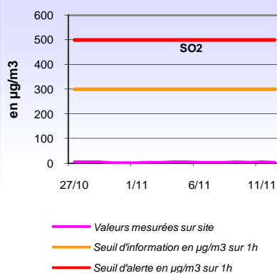
Evolution des maxima horaires en dioxyde de soufre
